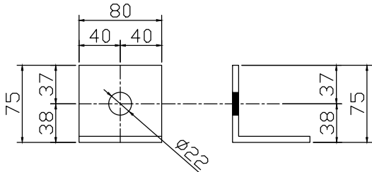
PEÇA A (FIXAÇÃO) CANTONEIRA L 3"x # 1/4" QUANTIDADE : 06 PÇS OBS: localizar pontos de fixação, e montar no fundo do painel.
